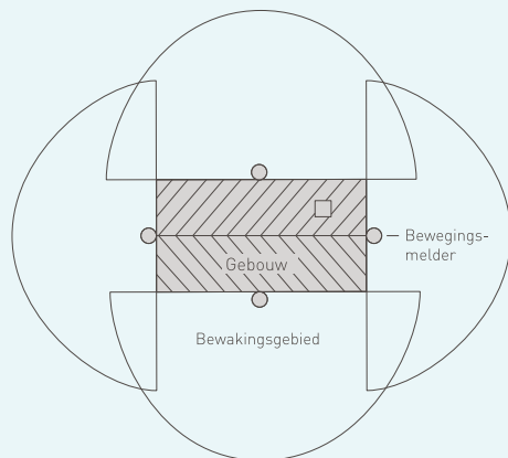
Omvangrijk bewakingsgebied bestaande uit vier eNet bewegingsmelders
