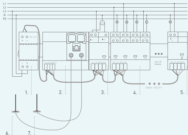
eNet DIN-rail-installatie met eNet server
