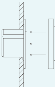
Installatietekening inbouwbasiselement
