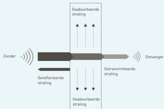
Reflectie, transmissie en absorptie van elektromagnetische straling
